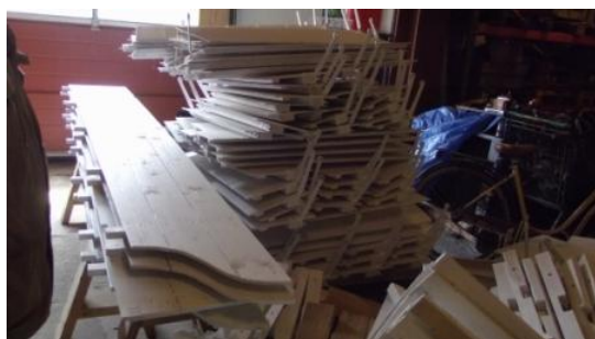
vindbrædder og lameller til Højsager Mølle
